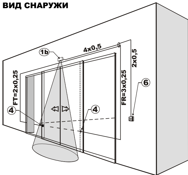
ВИД СНАРУЖИ
